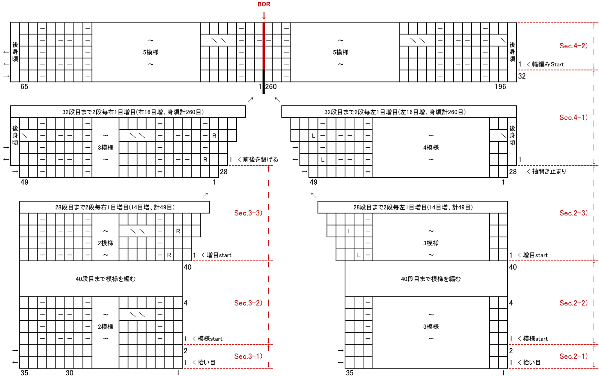
Chart3 : 左前身頃
